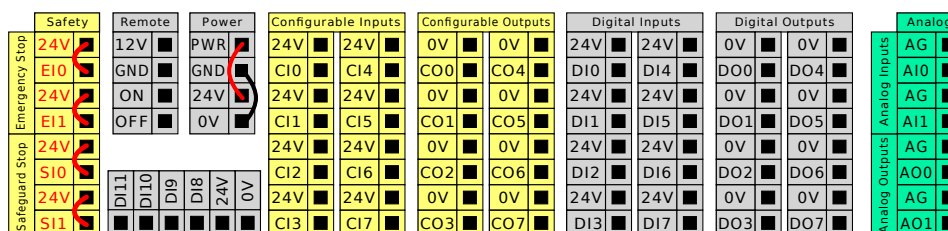
Skupine vhodov in izhodov (V/I).
