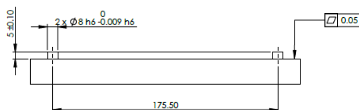
1.2: Płyta montażowa do podstawy robota
