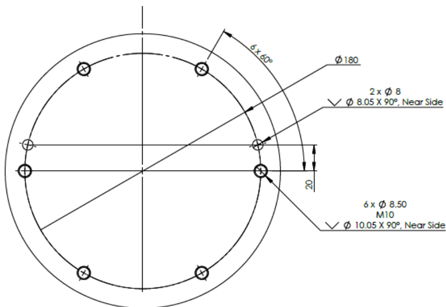
1.1: Vista dal basso della base del robot
