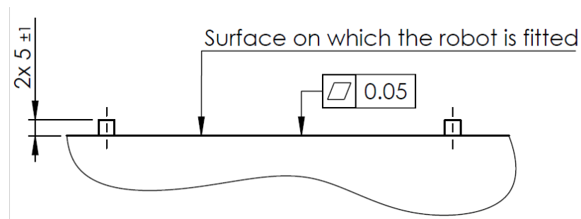
1.2: Piastra di montaggio per base robot
