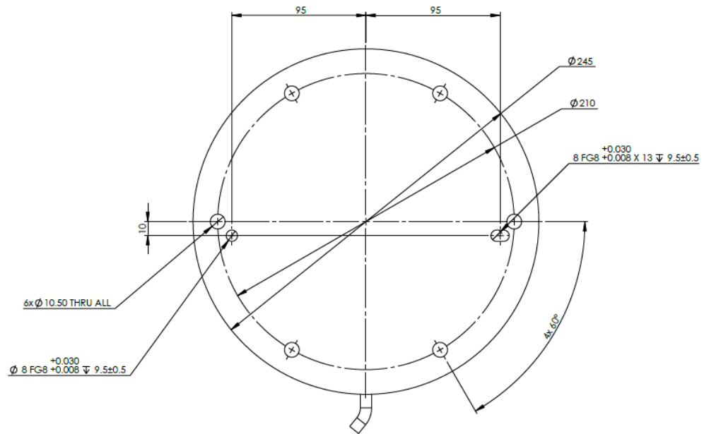
1.1: Vue de dessous de la base du robot
