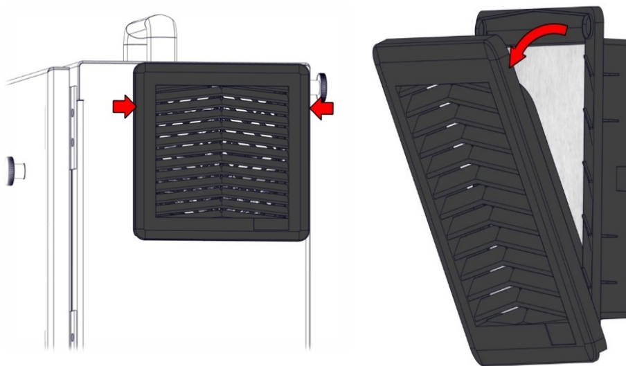
Figure 3.7. Remplacer les filtres du boîtier de commande.
