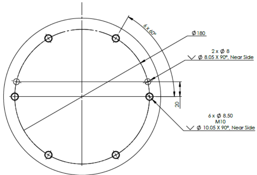
1.1: Vue de dessous de la base du robot
