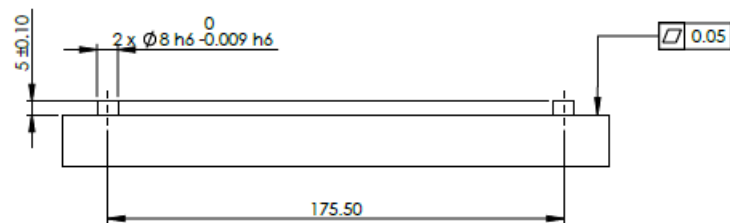
1.2: Plaque de montage pour base de robot
