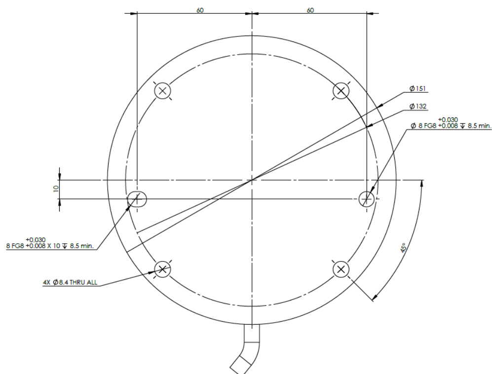
1.1: Ansicht der Roboterbasis von unten
