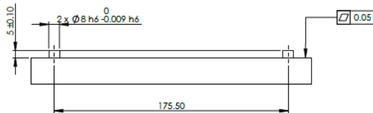
1.2: Montageplatte für Roboterbasis
