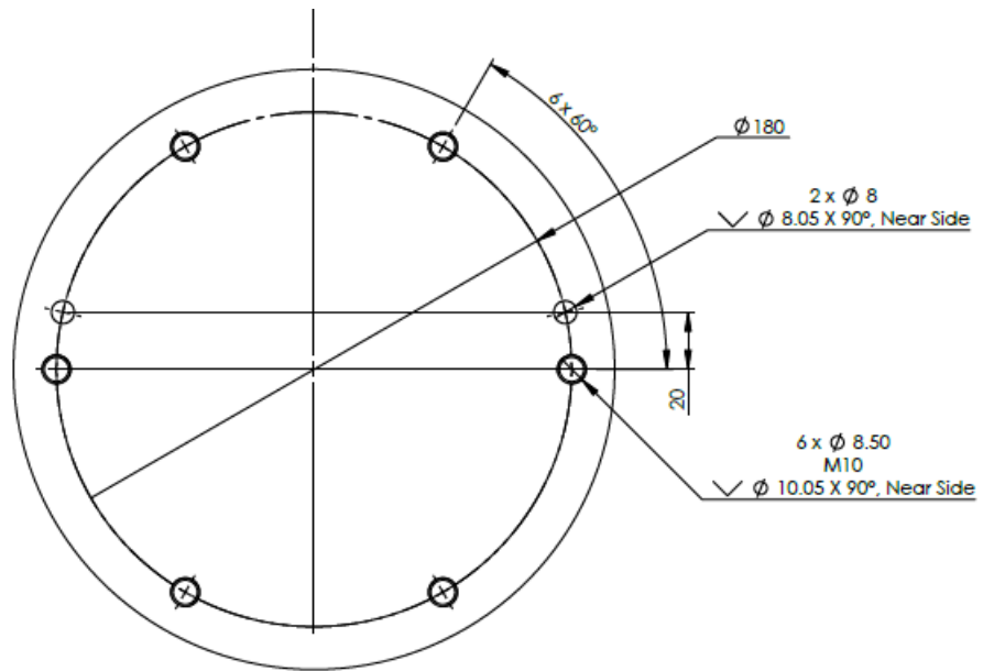
1.1: Ansicht der Roboterbasis von unten
