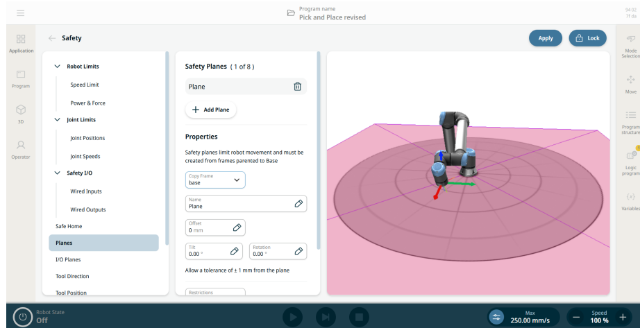
Abbildung 1.5: Bildschirm von PolyScope X, der Sicherheitsebenen anzeigt.
